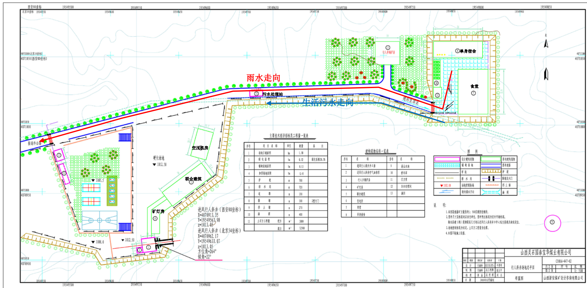
图 3 行人斜井场地总平面布置图 (应包括主要工序、厂房、设备位置关系,注明厂区雨水、污水收集和运输走向等内容)
