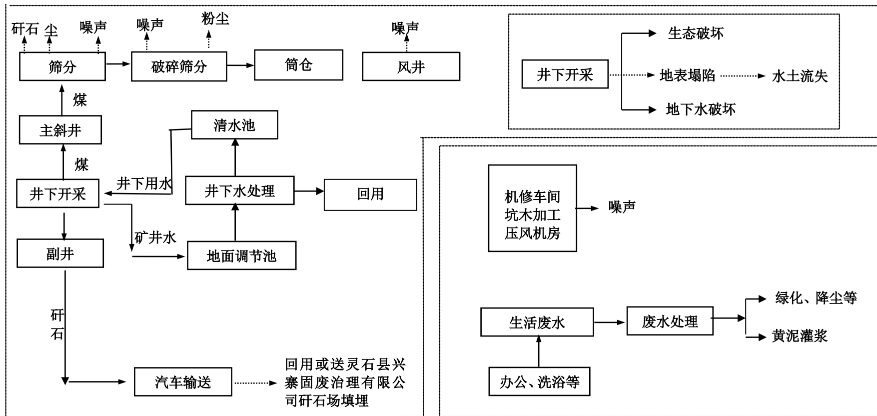
图1 生产工艺流程图 (应包括主要生产设施(设备)、主要原燃料的流向、生产工艺流程等内容)
